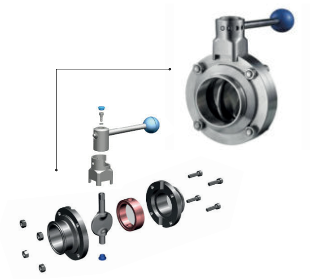
Válvula mariposa con manillar de palanca
